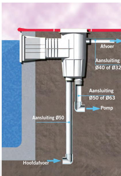
Installatie skimmer
