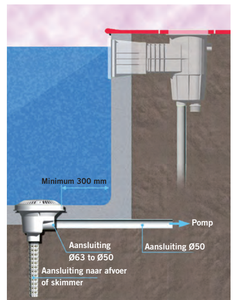
Installatie hoofdafvoer
