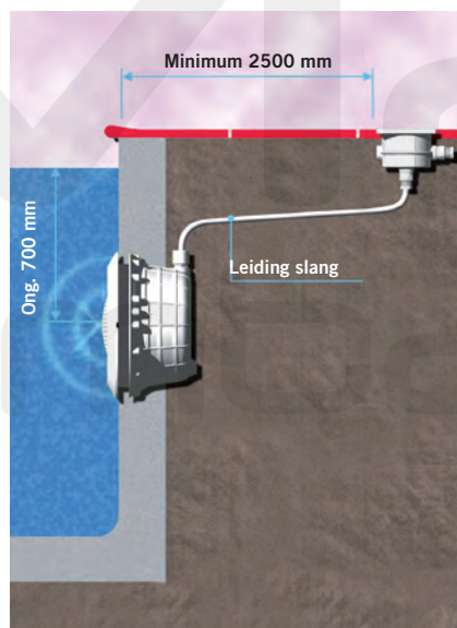
Onderwaterinstallatie
