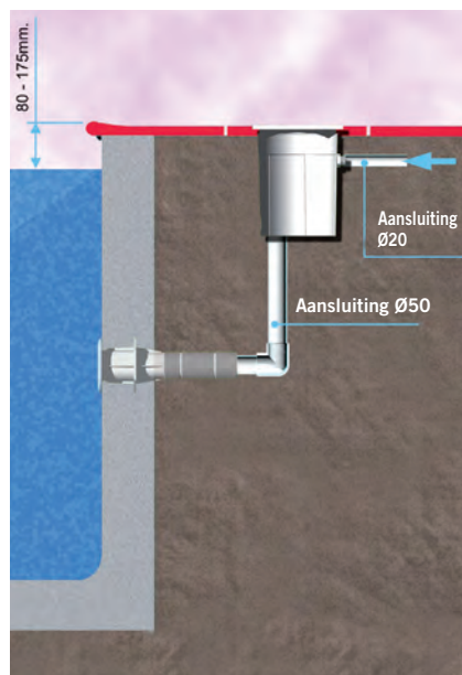
Installatie waterniveaugelaar
