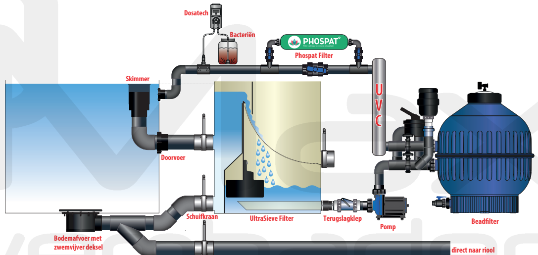
In deze filterinstallatie is een AquaForte UltraSieve gebruikt als voorfilter.
