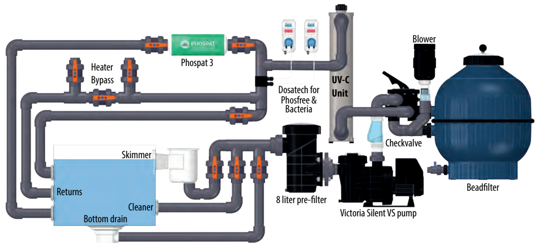
In deze bovengrondse filterinstallatie is een complete plug & swim pallet gebruikt.
