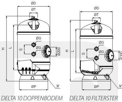
DELTA 10 DOPPENBODEM
